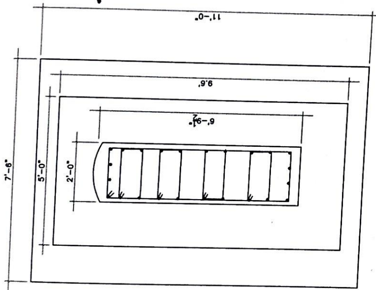
FB-PLAN
